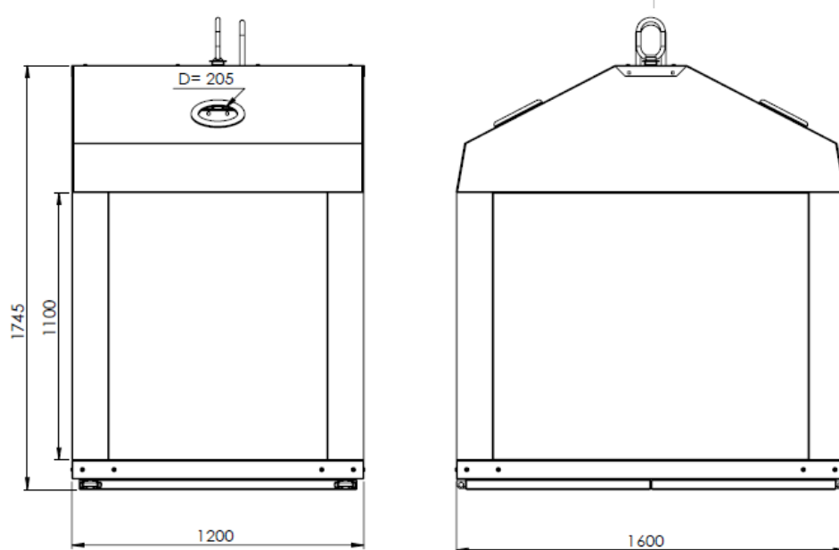
(Grundmaße Container)
