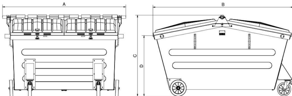
Abb. Mit Sonderausstattung „Verschlussblech“ und Kundenlogo seitlich
