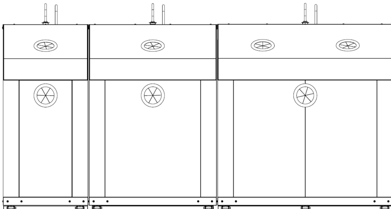
Depotcontainer 4.0m³, 1 Kammer, 3 Haken-Aufnahme mit einseitigem barrierefreiem Einwurf für alle Glasfraktionen
